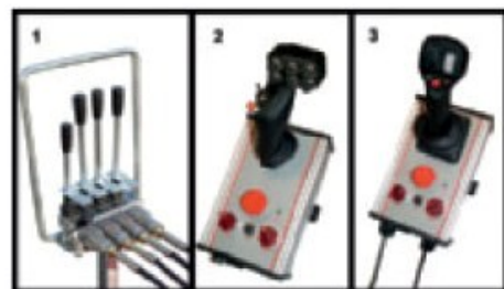
Verschillende bedieningsconsoles; 1 = teleflex kabels (standaard) / 2 = drukknoppen, elektrisch, z/w (optie) / 3 = joystick proportioneel (optie).
